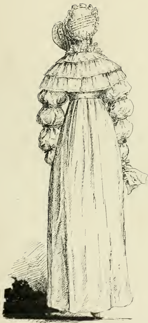
Fig 536. — Mode de 1815.
